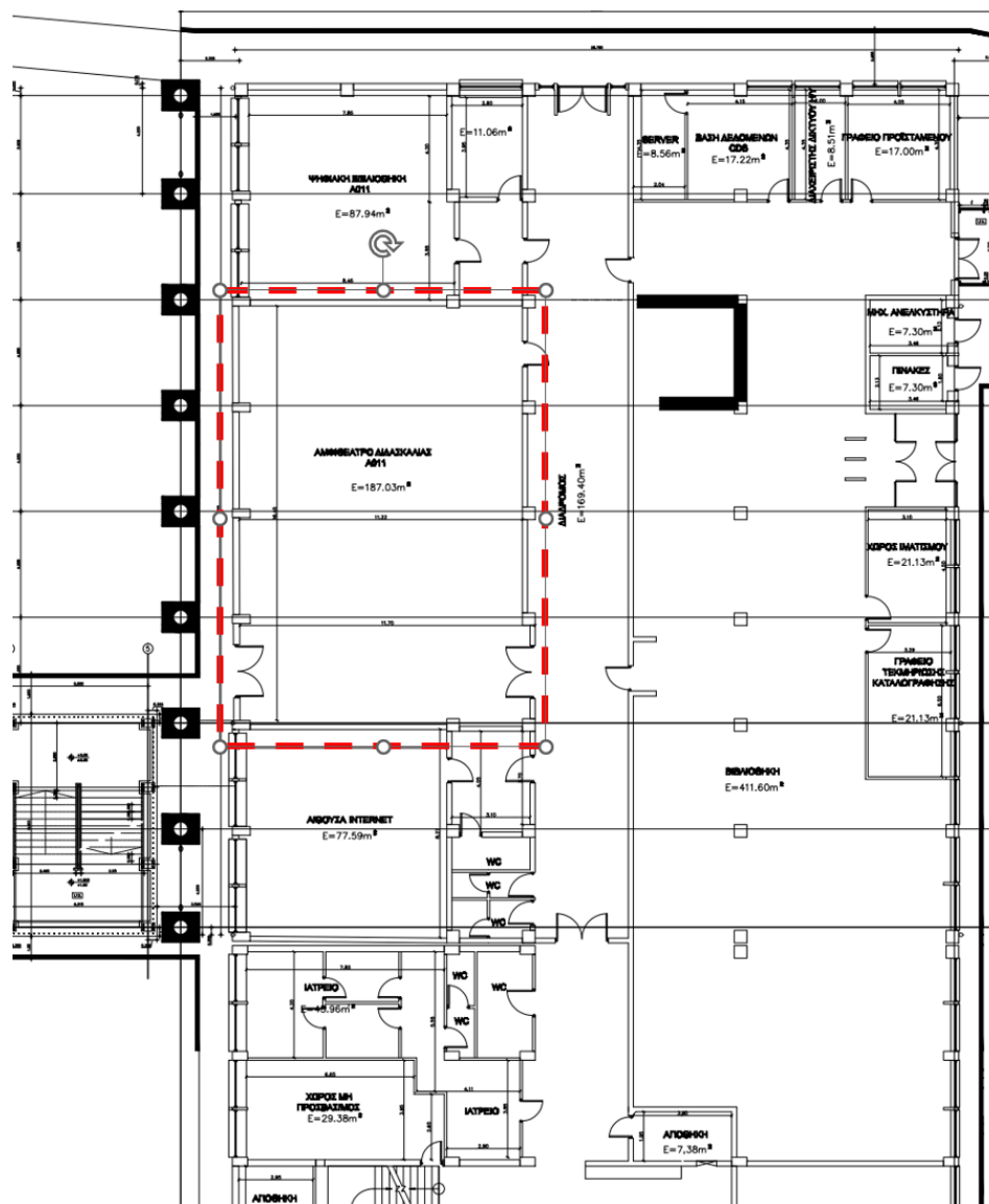
Εικόνα 5 Σχέδιο Αμφιθέατρου «Α011» - Κτίριο Βιβλιοθήκης
