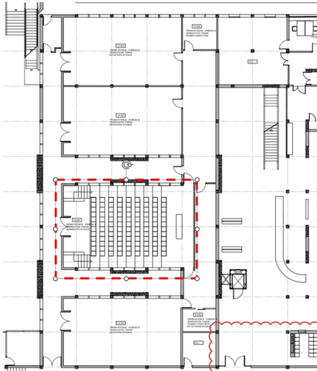
Εικόνα 2 1 Σχέδιο Αμφιθέατρον «Φυσικής» - Κτίριο Κ3
