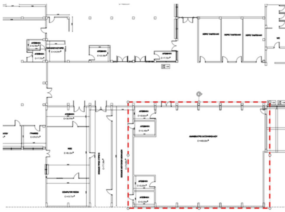
Εικόνα 4 Σχέδιο Αμφιθέατρου «Χατζηνικολάου» - Κτίριο Α
