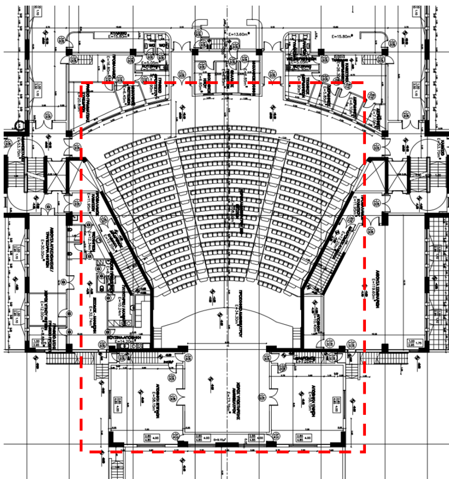
Εικόνα 6 Σχέδιο Αμφιθέατρου «Συνεδριακού Κέντρου» - Κτίριο Συνεδριακού Κέντρου
