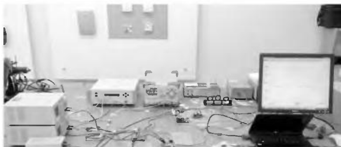
Το συμβολόμετρο, στηρίζεται στη διάδοση μιας μικροκυματικής συχνότητας μέσα σε μια οπτική ίνα κλειστού βρόχου
