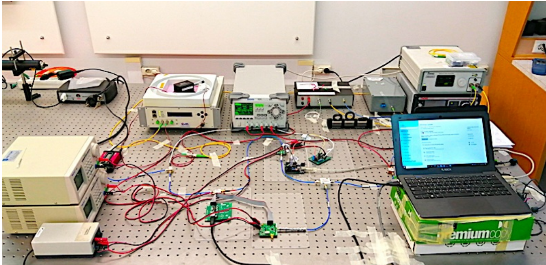
Σχήμα της πειραματικής διάταξης μέτρησης σεισμών MFFI που λειτουργήσε στα εργαστήρια του ΟΤΕ από τον Ιούλιο του 2021 έως τον Φεβρουάριο του 2022
